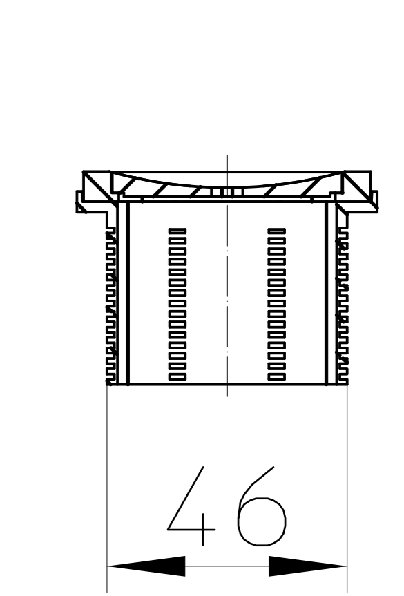
Schnitt B-B
